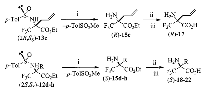
Scheme 9. Key: i) TFA, MeOH; ii) KOH 0.5 N, MeOH/ \text{H}_2\text{O} 7:3; iii) DOWEX-50 W
