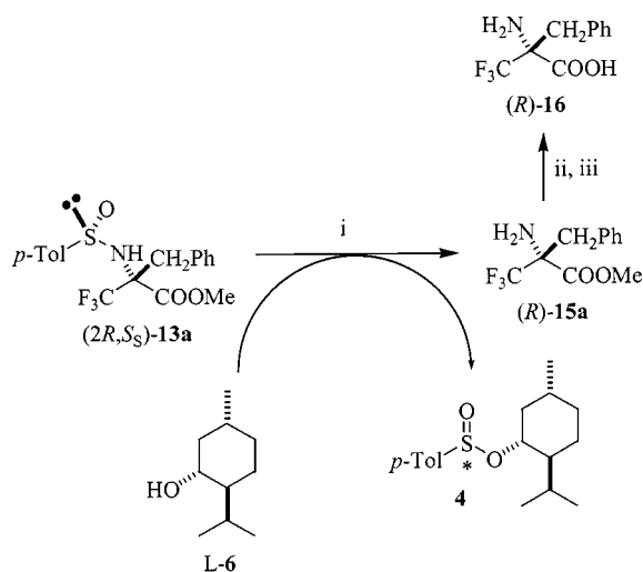
Scheme 8. Key: i) TFA, \text{CH}_2\text{Cl}_2 ; ii) KOH 0.5 N, MeOH/ \text{H}_2\text{O} 7:3; iii) DOWEX-50 W
